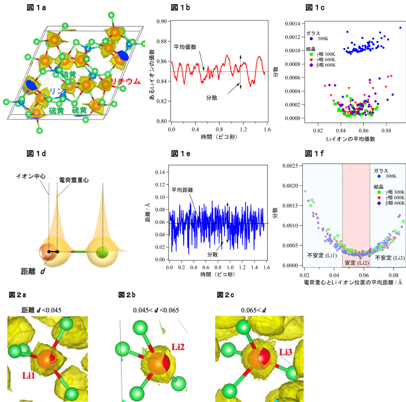
図1 : Bader 電荷分析法で評価した Li イオンの環境。(a) \text{Li}_2\text{S}-\text{P}_2\text{S}_5 結晶の Bader 法から得られた Li イオンの電荷密度。(b) Li イオンの 1.6ps の間の平均価数振動と分散。(c) ガラス相 ※10 、結晶 \beta 相、結晶 \gamma 相の Li イオンの平均価数と分散の相関。(d) Bader 解析で得られる距離情報。(e) 1.6ps 間の Li イオン位置と電荷雲重心の平均距離と分散。(f) ガラス相、結晶相各々の Li イオン位置と電荷雲重心の平均距離と分散の相関関係。
