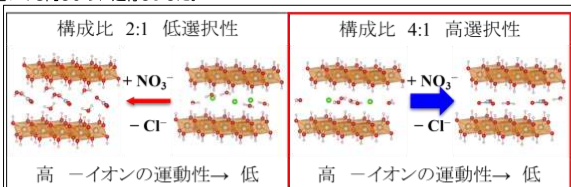
図2. 得られた精密結晶構造と選択性および層間の陰イオンの運動性の関係
